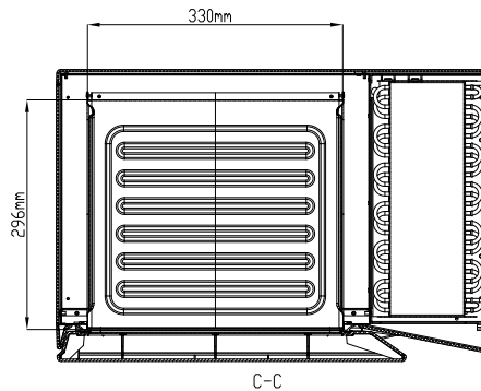
SEZIONE C-C C-C SECTION
