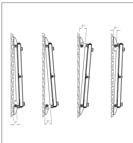
Neigungseinstellung (0° / ± 3° / ± 5°)
